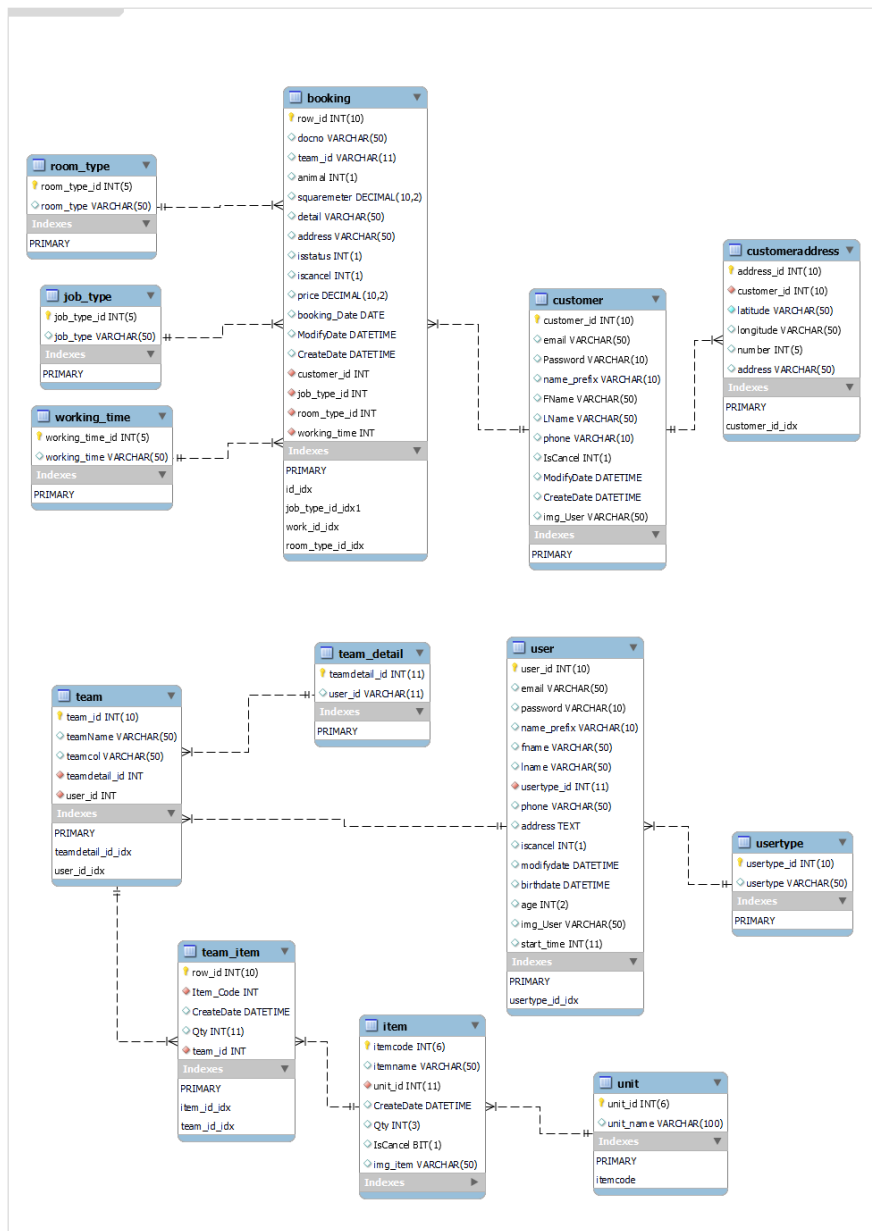
ภาพที่ 3.10 แสดงความสัมพันธ์ข้อมูล (ER-Diagram)
