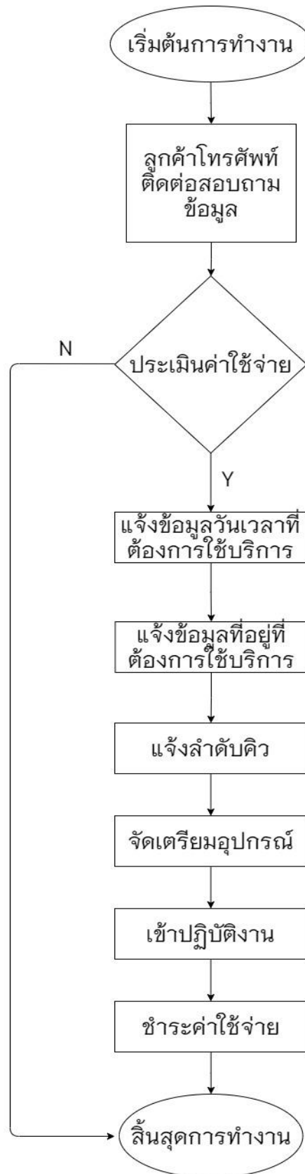
ภาพที่ 3.2 แสดงแผนผังการทำงานในระบบงานเดิม
